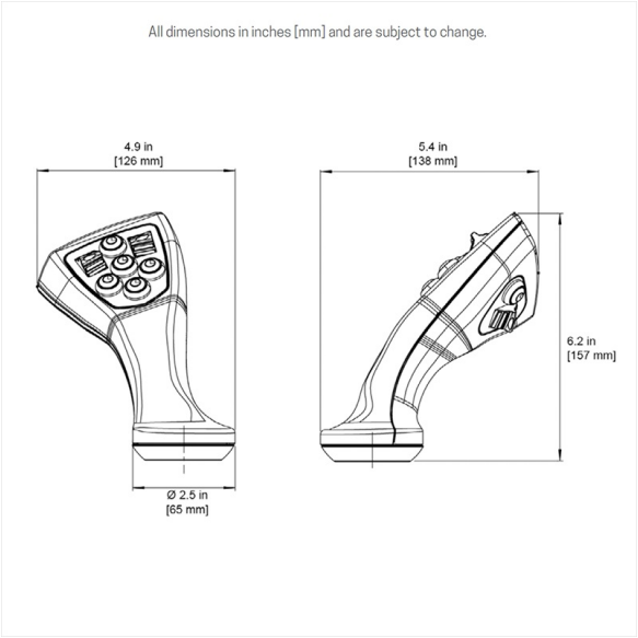
G56 dimensions
