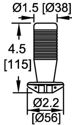
RH dimensions
